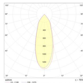
Krzywa rozsyłu 38°
