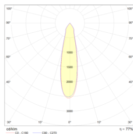
Krzywa rozsyłu 24°
